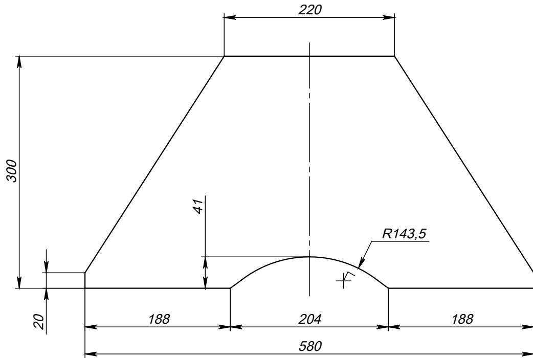
Поз.1 (Корпус) развертка
